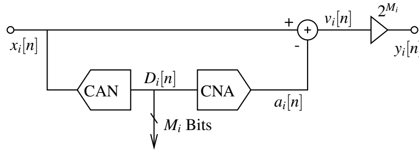
FIGURE 1.3 – Schéma bloc d'un étage Pipeline
